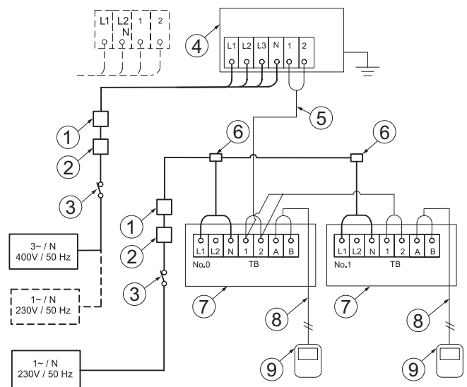
Alimentation électrique indépendante du groupe extérieur et de l'unité intérieure
