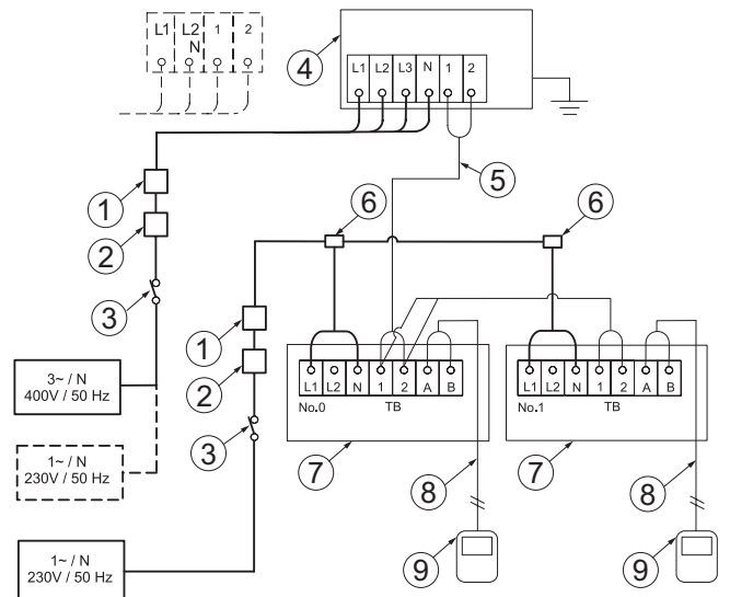
Fuente de alimentación independiente de la unidad exterior y la unidad interior
