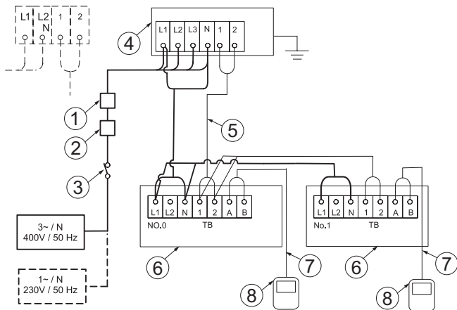
Alimentation du groupe extérieur à l'unité intérieure
