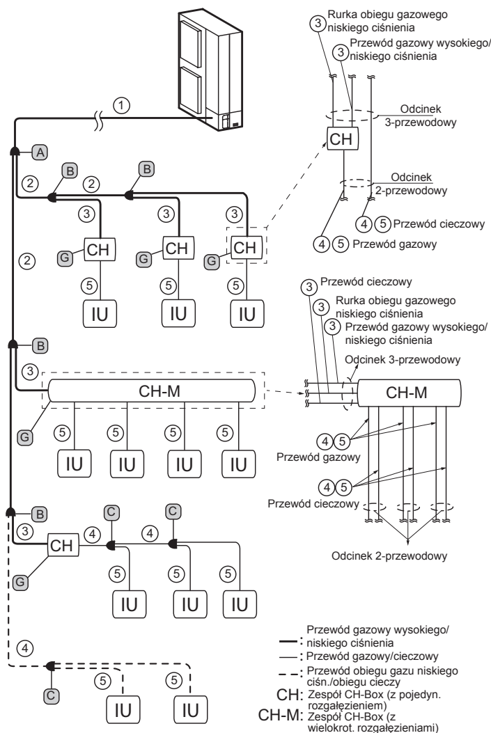
Kolektor rozgałęźny zastosowany w miejsce zestawu Multi-Kit:
