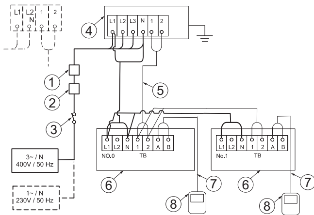
Alimentación desde la unidad exterior a la interior
