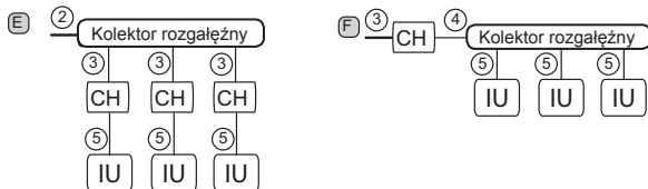
Kolektor rozgałęźny zastosowany w miejsce zestawu Multi-Kit:
